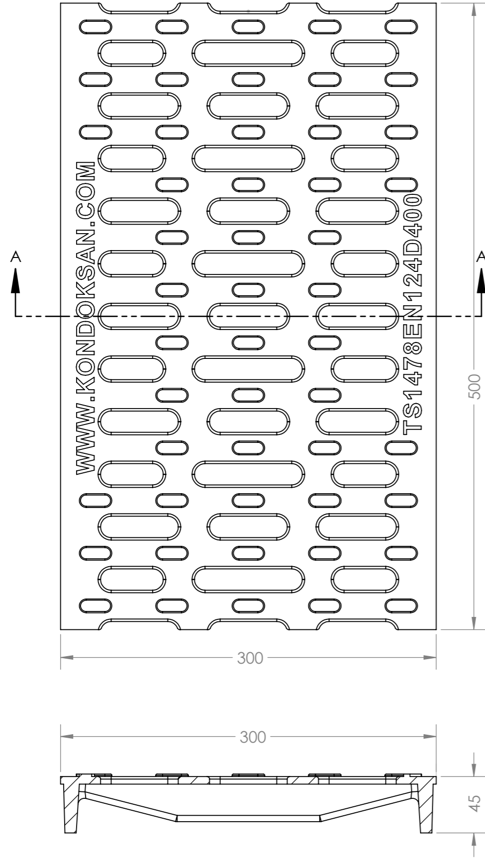
KESIT A-A ÖLÇEK 1 : 3
