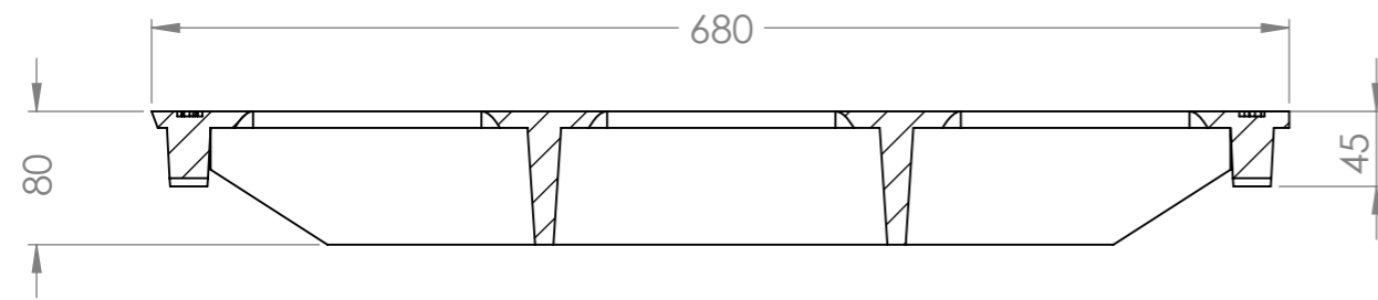
KESIT AD-AD
