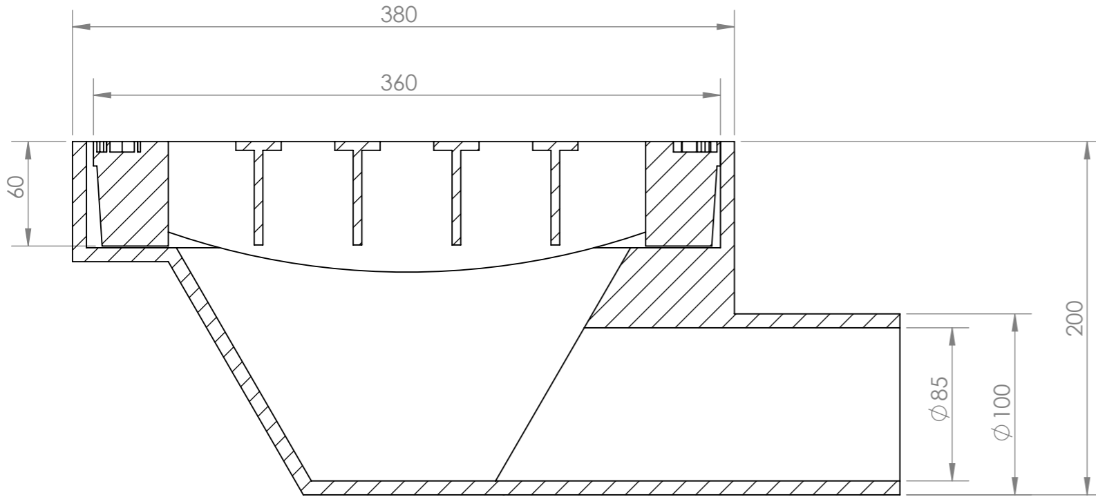
KESIT B-B ÖLÇEK 1 : 3
