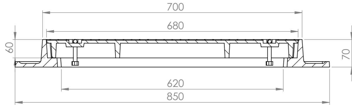
KESIT A-A ÖLÇEK 1 : 6
